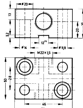
SDA-22x1,5-B
