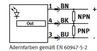
Adernfarben gemäß EN 60947-5-2
