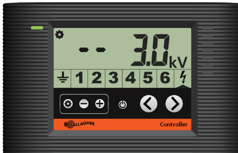
Bedieningspaneel toont de standaard schrikdraadapparaataalarminstellingen met stroomsterkte uitgeschakeld en spanning op 3.0KV
