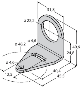
montagebeugel, roestvaststaal, voor bouwworm K30L
