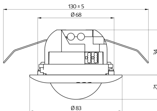
Afmetingen 93360
