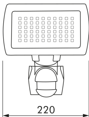
Afmetingen 92627
