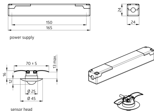
Afmetingen 92910
