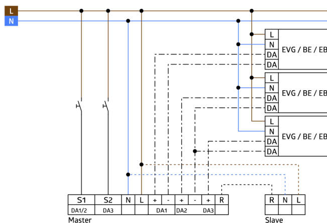
Schakelschema
