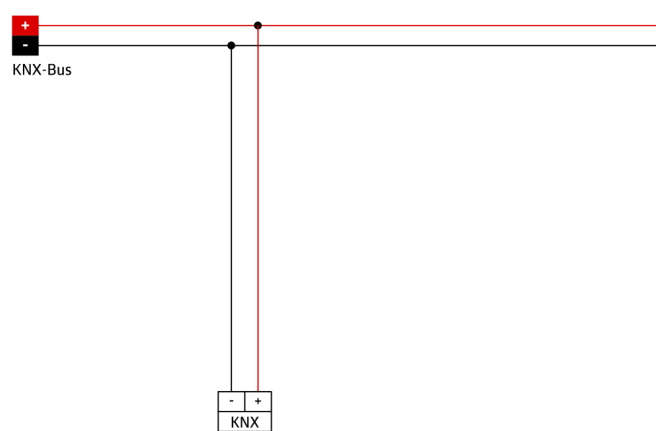
Schakelschema
