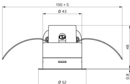
Afmetingen 93392
