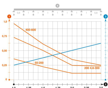
Belastingsdiagram draadgoot GR-Magic type GRM 55
