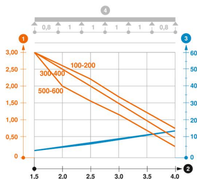
Belastingsdiagram kabelgoot type SKSM 110
