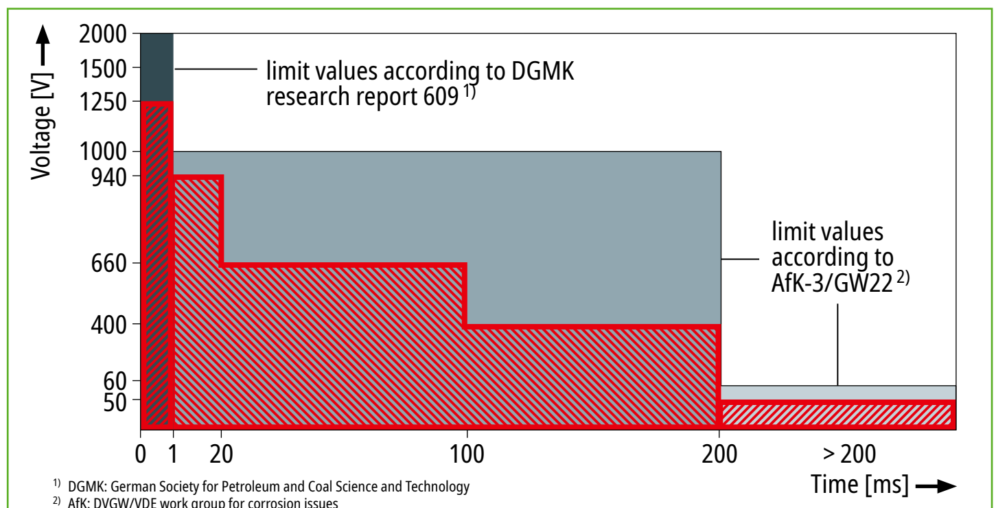
Fig. 1 Voltage limit values
