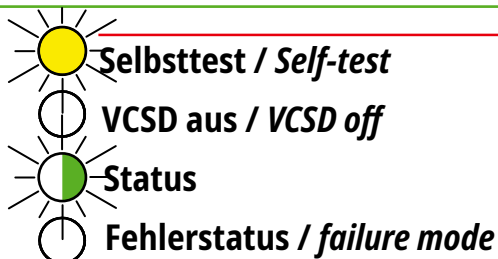
Fig. 4.2h „Selbsttest“ LED-Anzeige
