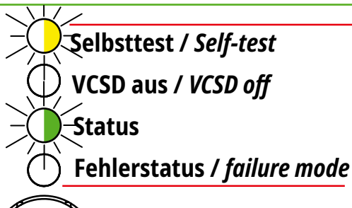
Fig. 4.2f „Selbsttest“ LED-Anzeige
