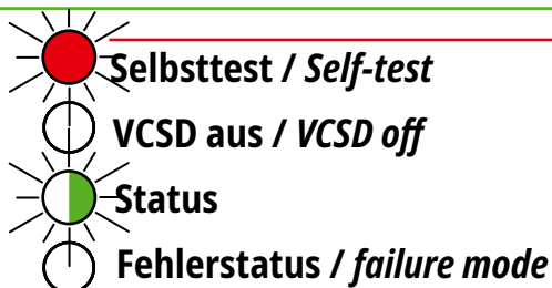
Fig. 4.2i „Selbsttest“ LED-Anzeige
