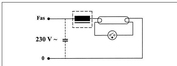
Starter enkelvoudige aansturing (inductief)
