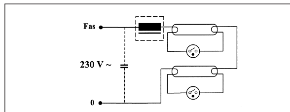
Starter serie aansluiting
