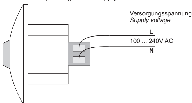
SR-MDS Netzspannung / Mains Supply
