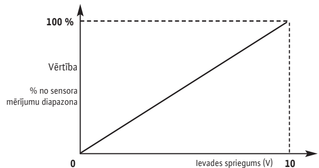
Sensora signāls 0–10 V
