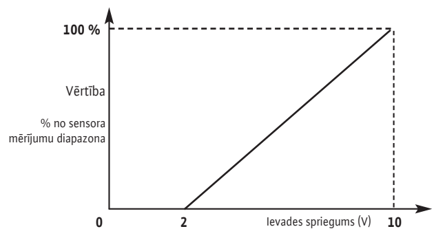
Sensora signāls 2–10 V
