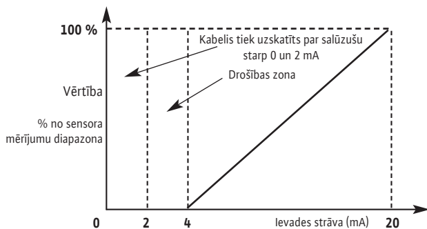
Sensora signāls 4–20 mA
