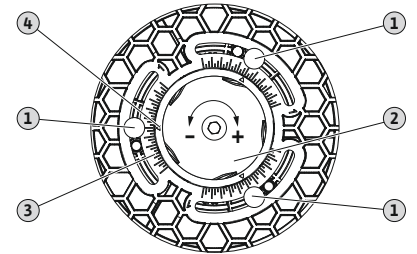
Fig. 8: إعادة ضبط فجوة العجلة الدافعة (المصفاة مفكوكة)
