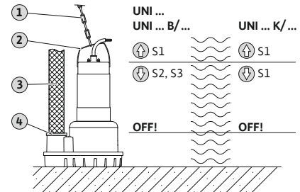
Fig. 3: التركيب المغمور، قابل للنقل
