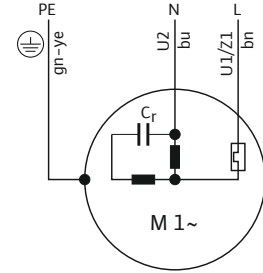
Fig. 4: مخطط التوصيل، محرك 1 ~
