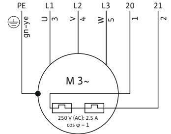
Fig. 5: مخطط التوصيل، محرك 3 ~
