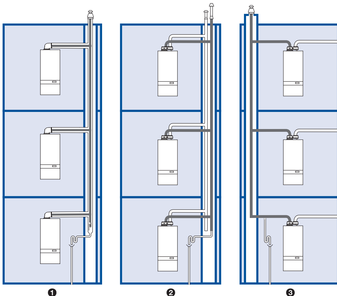
Uitvoeringen CLV overdruksystemen: 1 Concentrisch; 2 Parallel; 3 half CLV.
