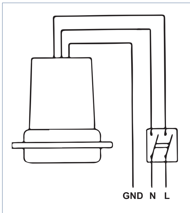
Aansluitschema
