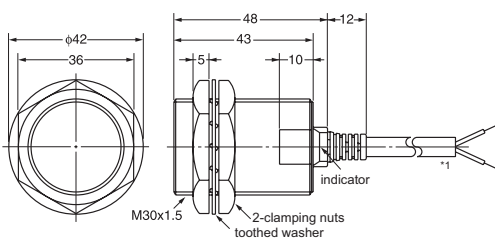
Fig. ⑦ E2AG-M30KS10-WS-B
