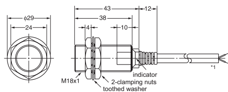
Fig. ⑤ E2AG-M18KS05-WS-B
