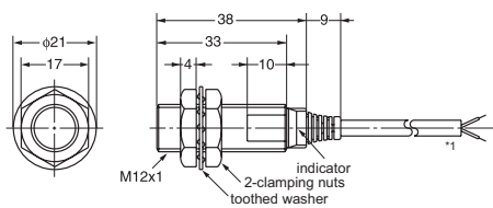
Fig. ③ E2AG-M12KS02-WP-B
