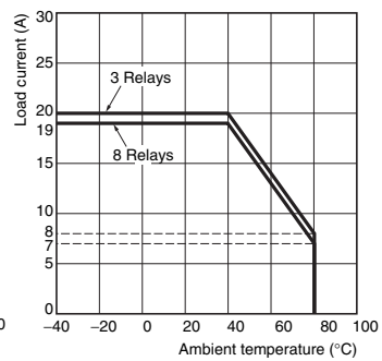
G3PE-525B(L)
