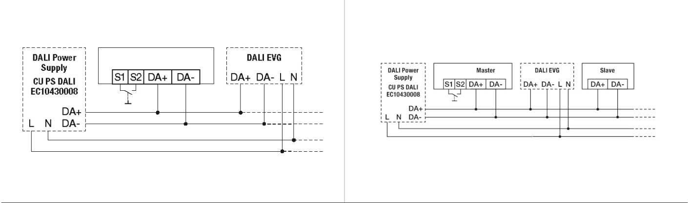
Standaardschema
