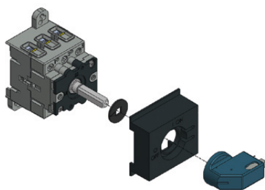
SIRCO MC PV Montage sur rail DIN
