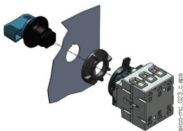
SIRCO MC PV Montage sur porte
