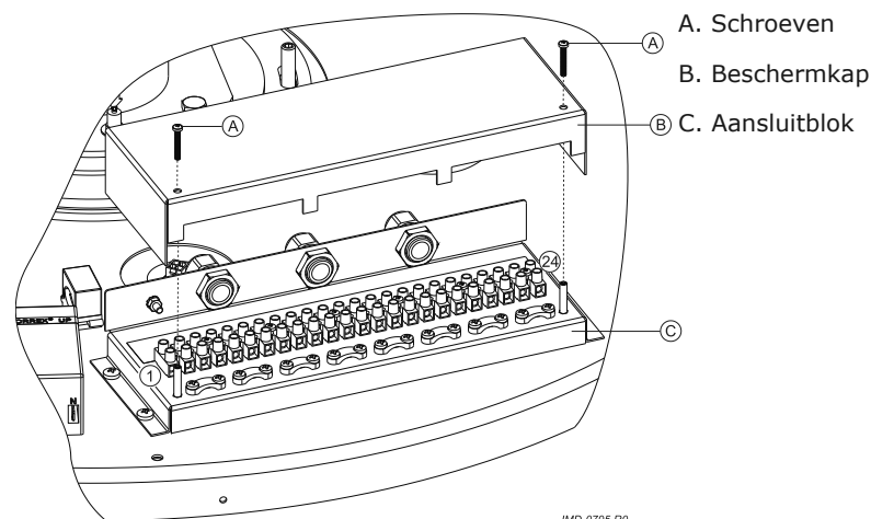
Afb. Aansluitingenblok
