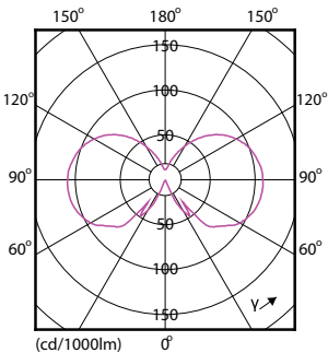
CLA LEDbulb 60W E27 840 CL A60
