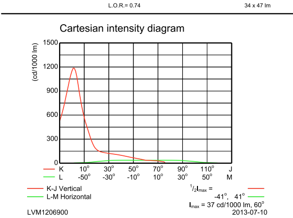
BBP623 GC 34xLED-HB/BL A
