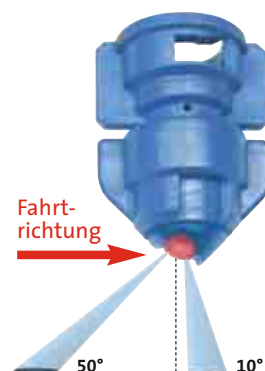
Asymmetrische Doppel-Flachstrahl-Injektordüse in Keramik
