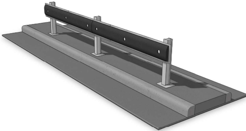
Verschraubung des Rammschutz.
